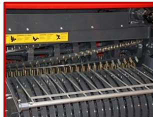
ระบบสับและเก็บด้ายแบบกว้าง WIDE CHOPPING AND COLLECTION SYSTEM
