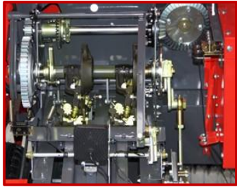
เครื่องผูกด้าย 2 ชุด 2 THREAD KNOTTER GROUP
