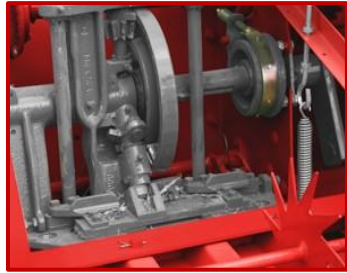
ชุดผูกปมร้อยสาย WIRED KNOTTER GROUP
