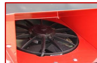
ชุดพัดลมทำความสะอาดกลุ่มเครื่องผูกปม KNOTTER GROUP CLEANING FAN
